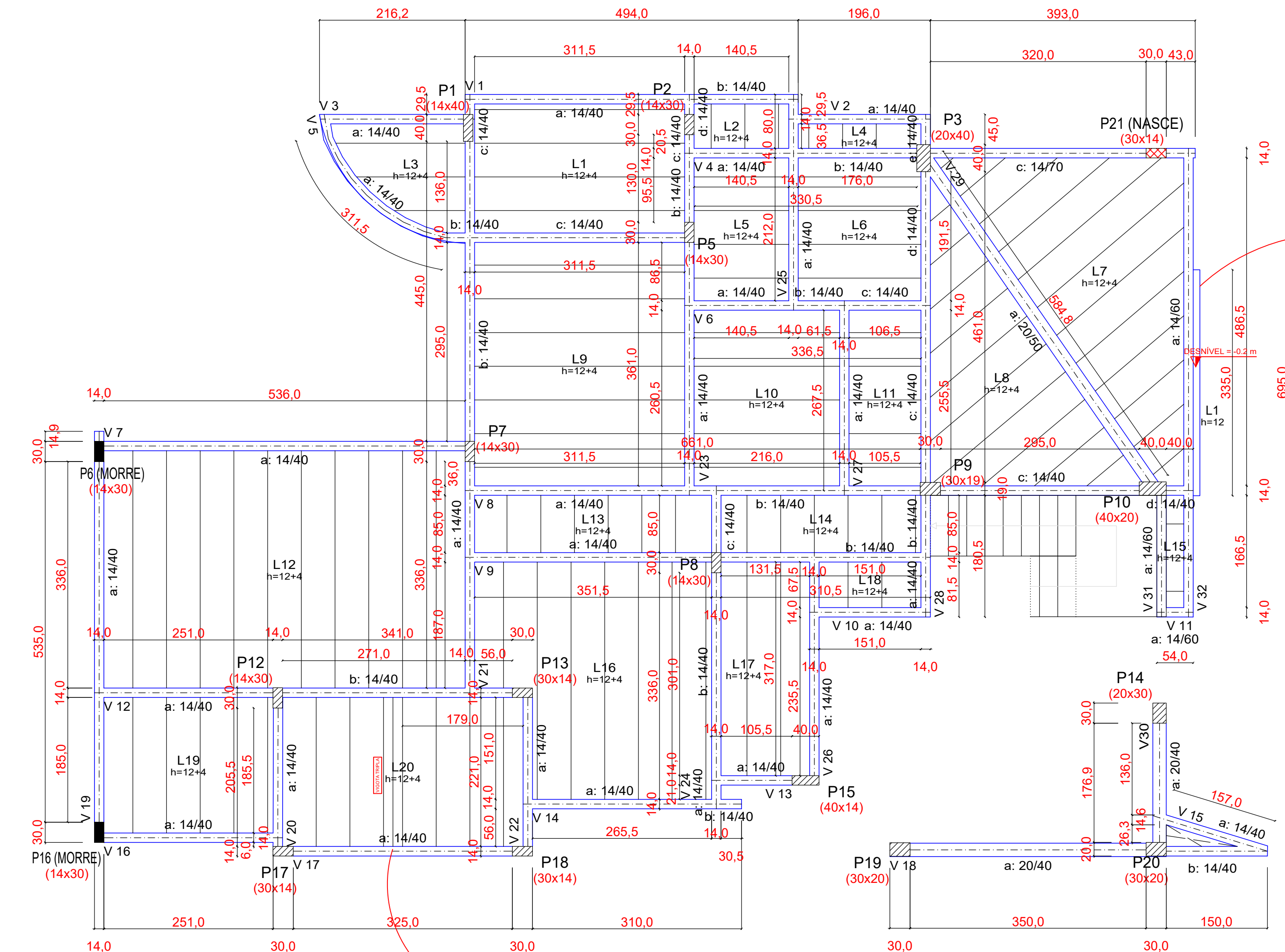
PLANTA DE FÔRMA - 1º ANDAR (+3,45) esc 1:50
